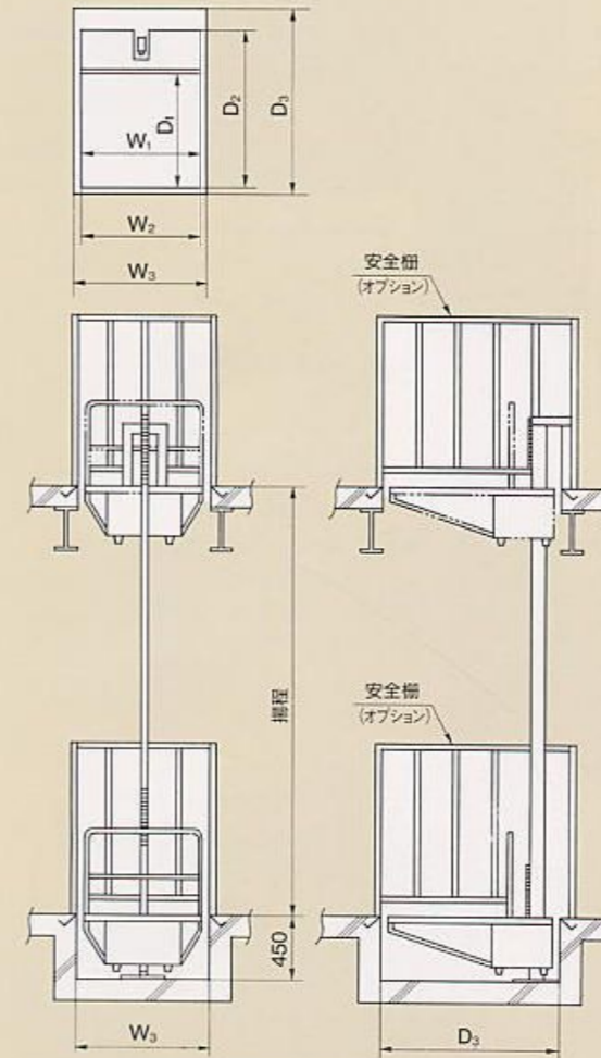
YV-2型、4型の安全柵及び両開き扉付寸法図
