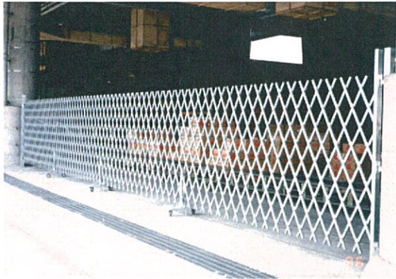
ロングドアLL 14.0m (Wキースタ-仕様・本設柱に取付)
